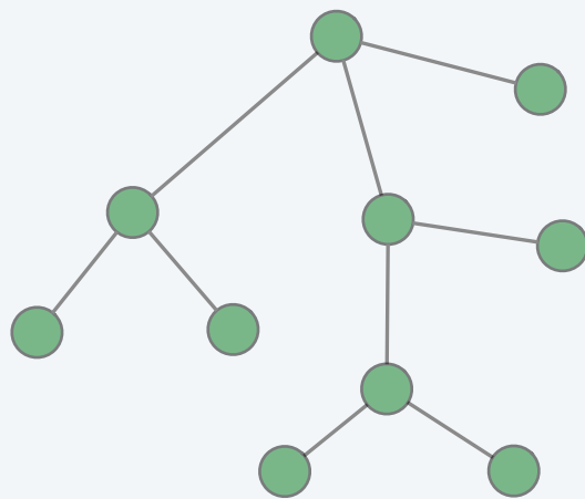
albero
