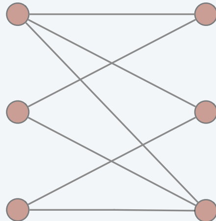
grafo bipartito
