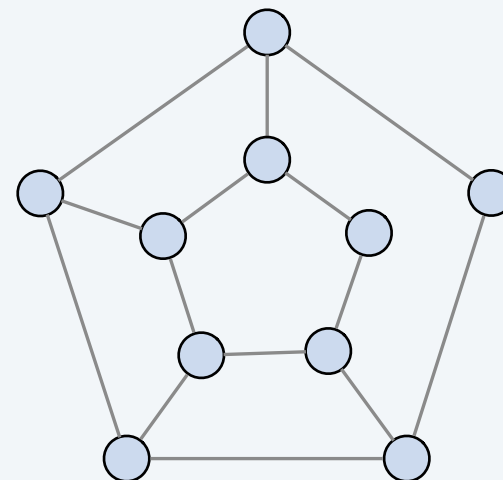
grafo planare
